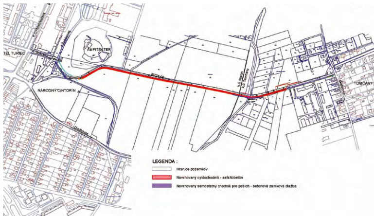
Schéma cyklotrasy a chodníka z Martina do Tomčian
